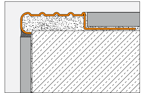
Variante de mise en œuvre de Schlüter®-TREP-E
