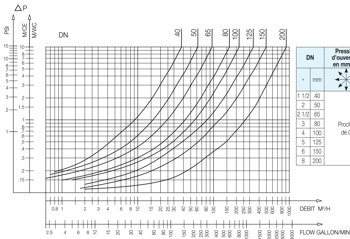
407 - Abaque des pertes de charge
